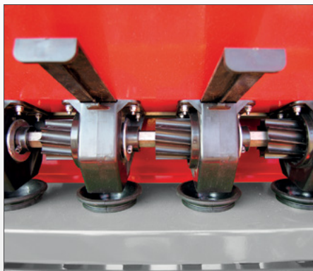
Висіваючий апарат для насіння
