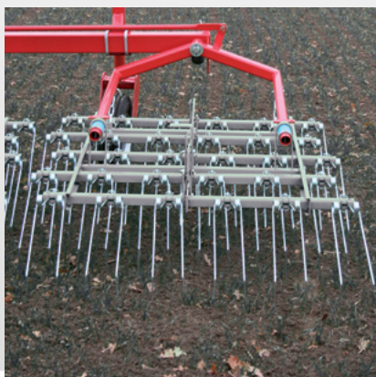
Робоча секція завдяки конструкції підвіски прекрасно копіює рельєф поля
