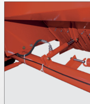
Гідравлічне регулювання підбирача (опція) - дозволяє управляти підбирачем з кабіни трактора
